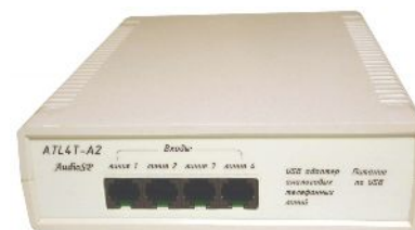
Рис. Вид спереди, входные розетки RJ11 – 4шт.
